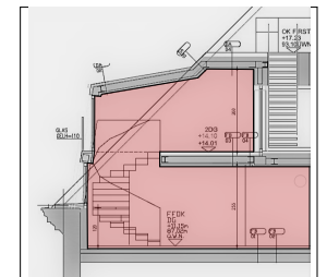
Schnitt A-A
