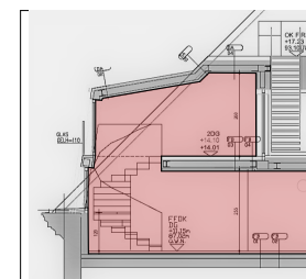
Schnitt A-A
