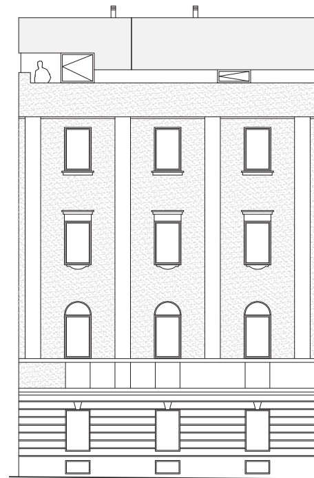
ansicht ost
