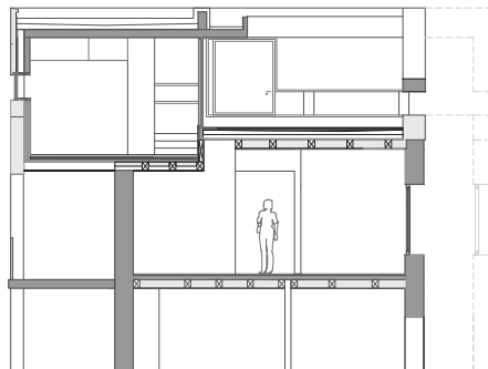
schnitt b_b
